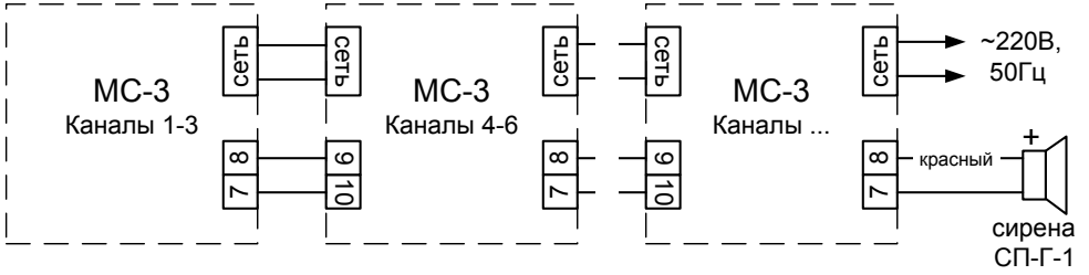
Рисунок А.6 – Схема соединения нескольких приборов MC-3 для работы с одной сиреной и подключения к общему электропитанию
